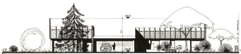
FAÇADE SUD. EST
